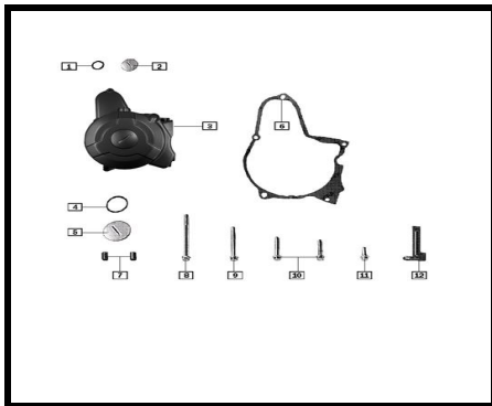
E-9 TAPA VOLANTE
