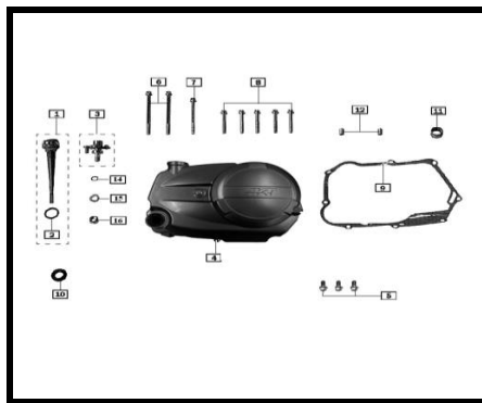
E-10 GENERADOR
