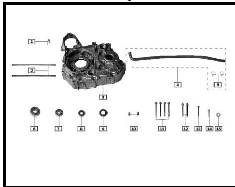
E-12 CARCAZA IZQUIERDA
