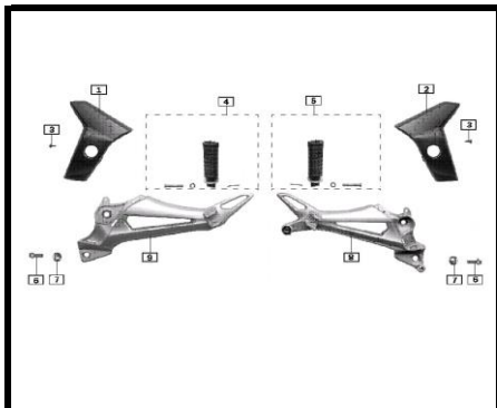
F-27 POSAPIES TRASEROS
