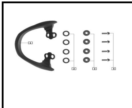
F-24 PARRILLA
