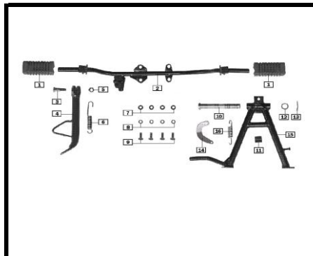
F-28 POSAPIE DELANTEROS
