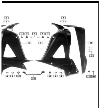
GUARDAPIERNAS
