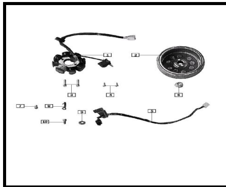
E-10 GENERADOR
