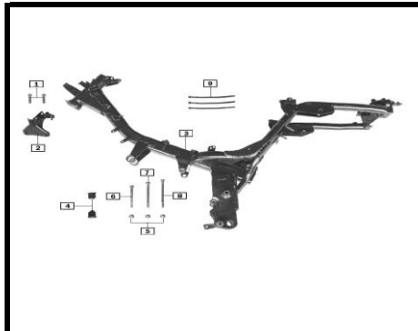
F-30 CHASIS
