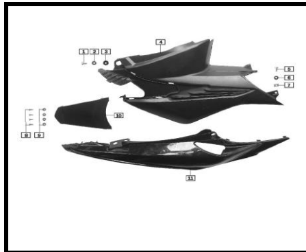
F-32 CARENAJE TRASERO DER
