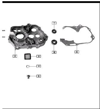
CARCAZA DERECHA
