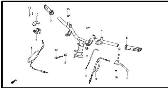
F- 5 CARENAJES MANUBRIO
