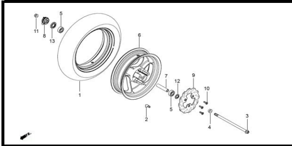
F-10 RUEDA DELANTERA
