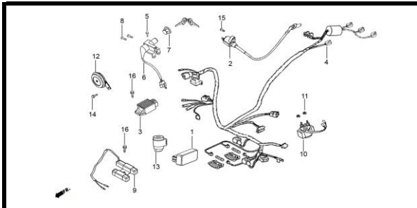
F-20 SISTEMA ELECTRICO
