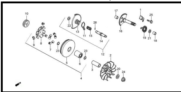
E-14 CAJA TRANSMISIÓN
